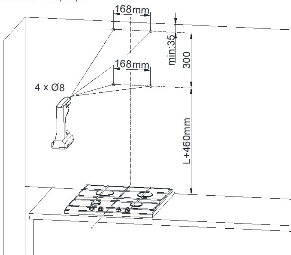
Рис. 5 Установочные размеры
