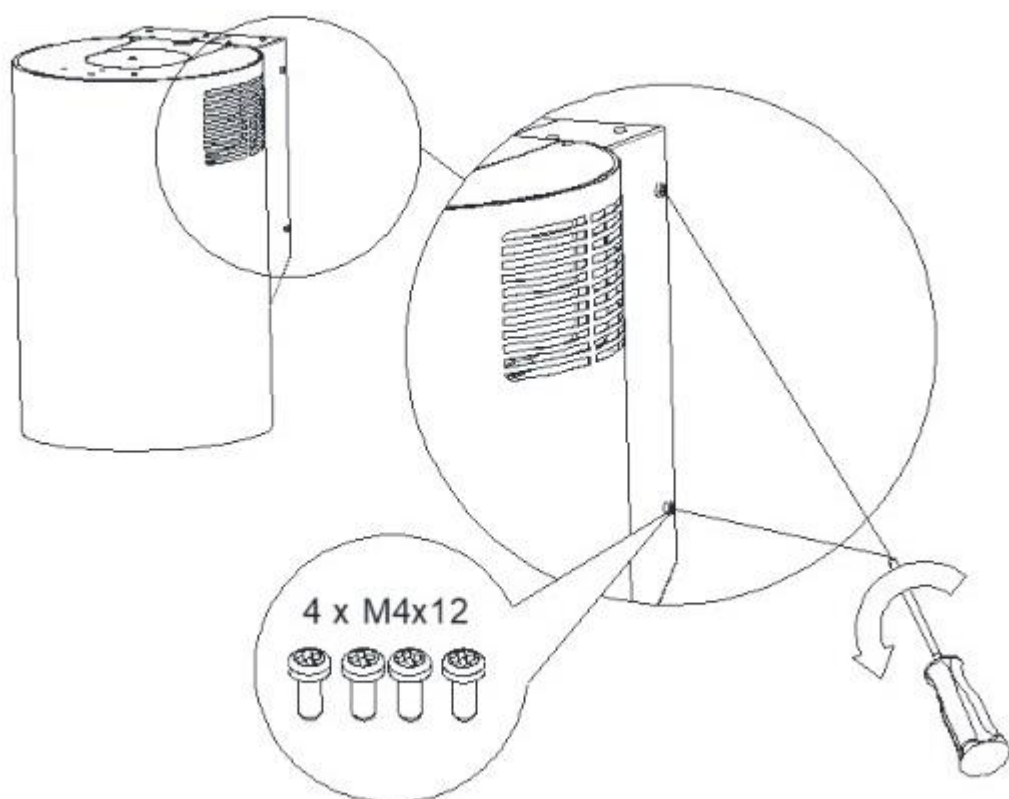
Рис. 7 Демонтаж держателя крепления вытяжки
