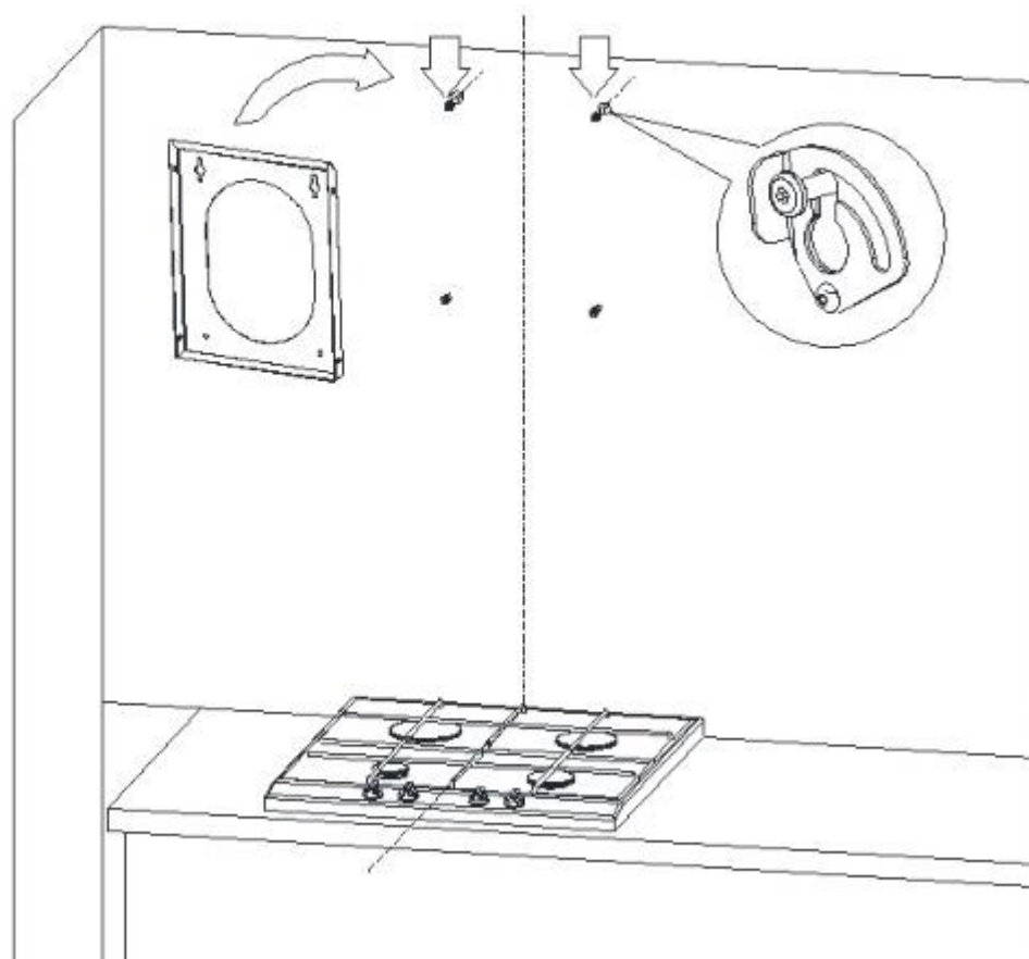
Рис. 8 Подвесной держатель для крепления вытяжки
