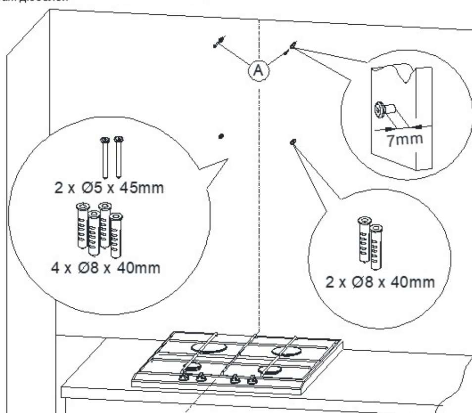
Рис. 6 Монтаж дюбелей
